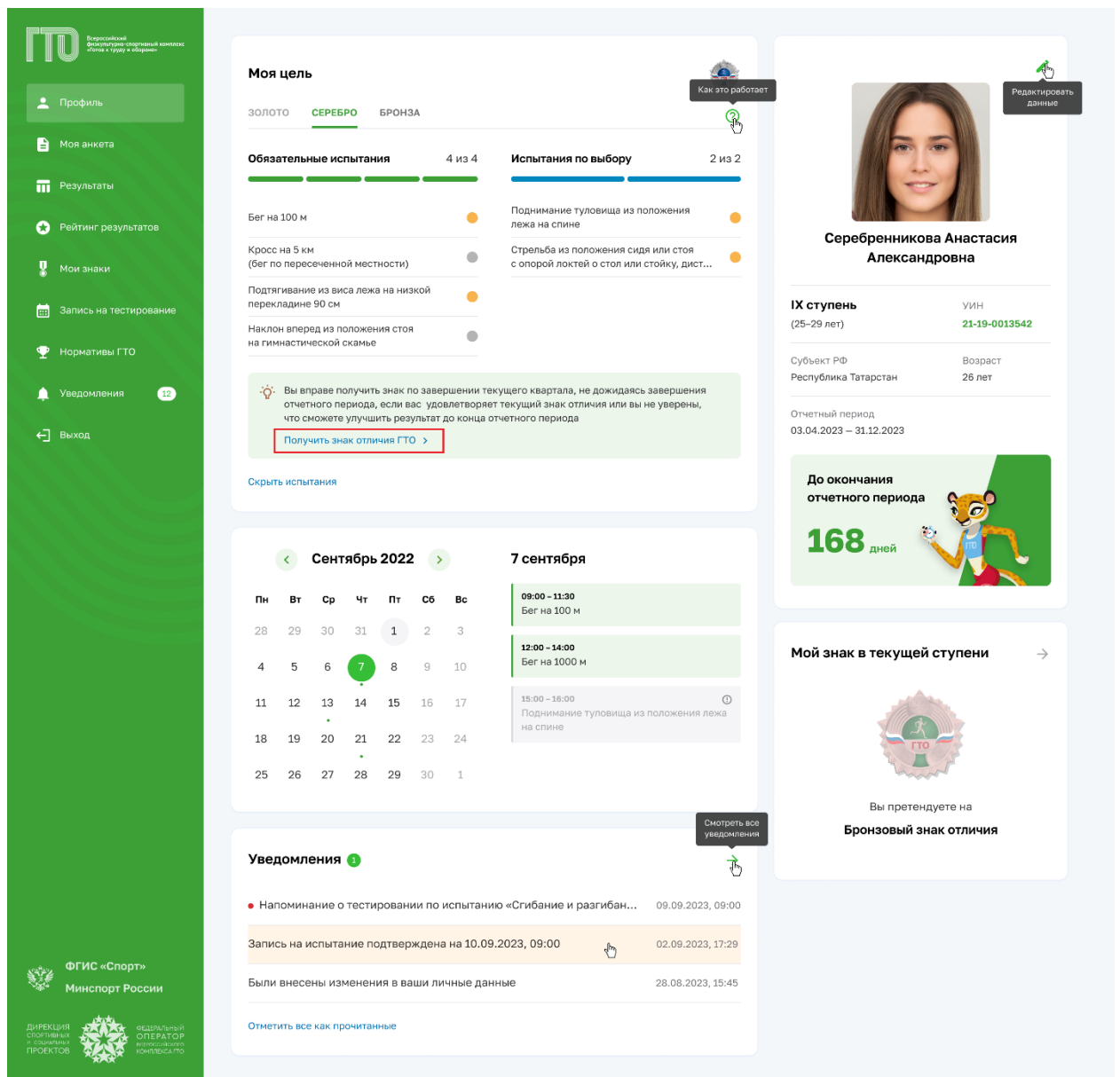
Рисунок 25. Страница «Профиль»
